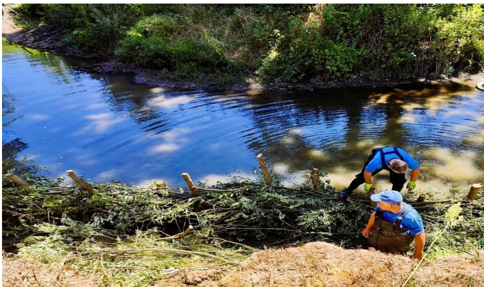
Consolidare vegetativă a râului Barcău, județul Bihor (Sursa foto: ABA Crișuri)
