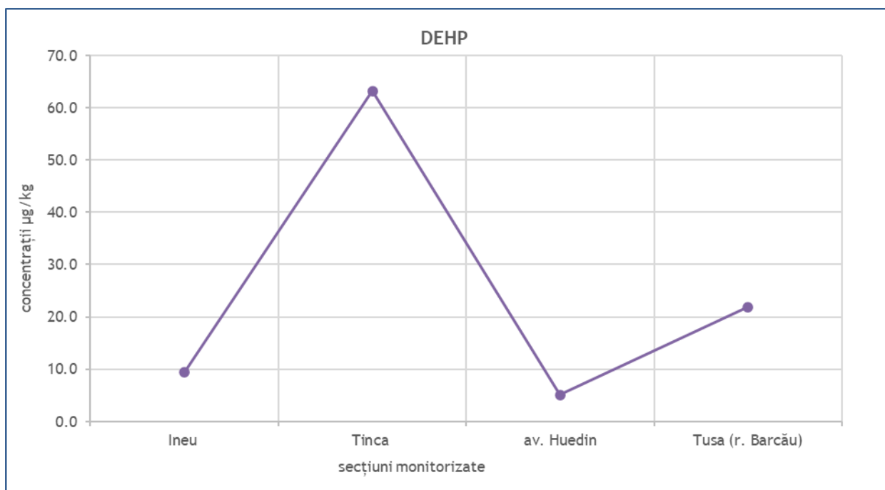
Figura 17 : Variația rezultatelor pentru DEHP în secțiunile monitorizate
