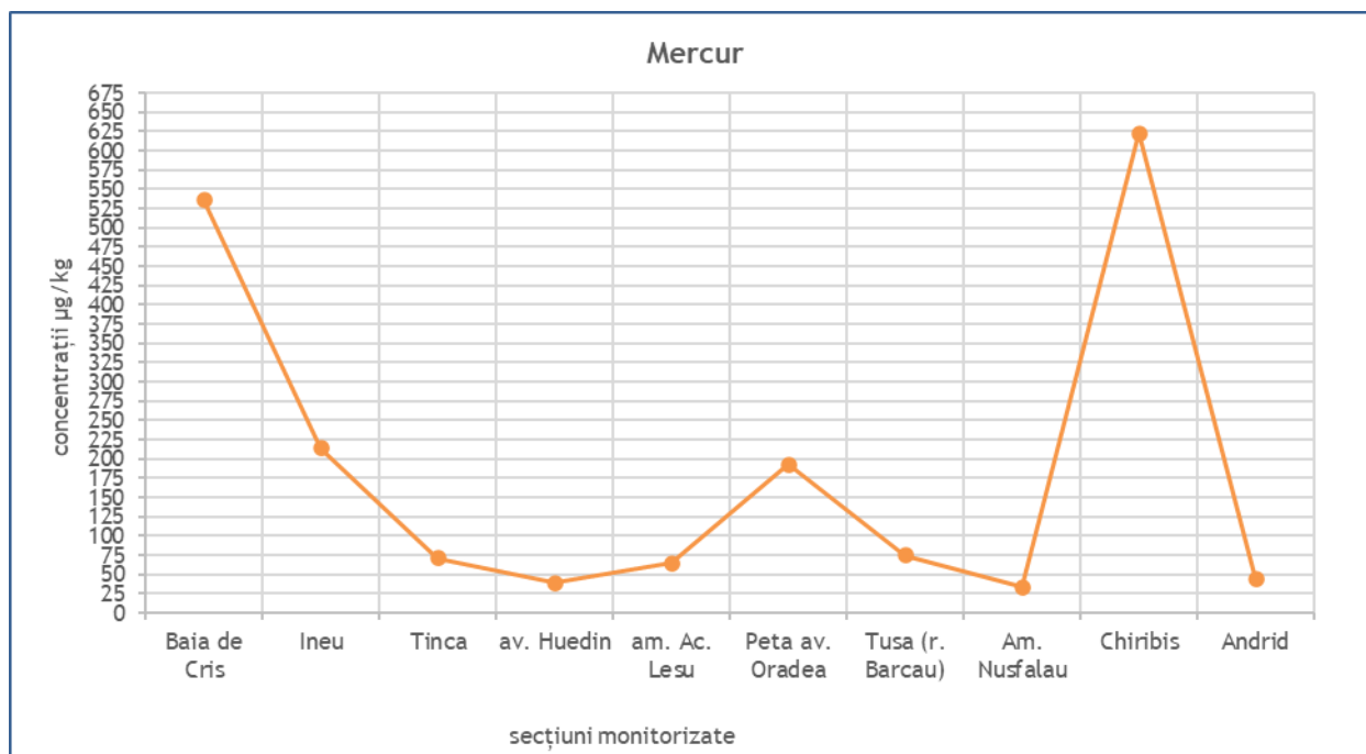
Figura 15 : Variația rezultatelor pentru Mercur în secțiunile monitorizate
