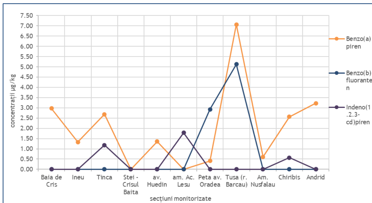
Figura 12 : Variația rezultatelor pentru benzo(a)piren, benzo(b)fluoranten, indeno(1,2,3-cd)piren în secțiunile monitorizate
