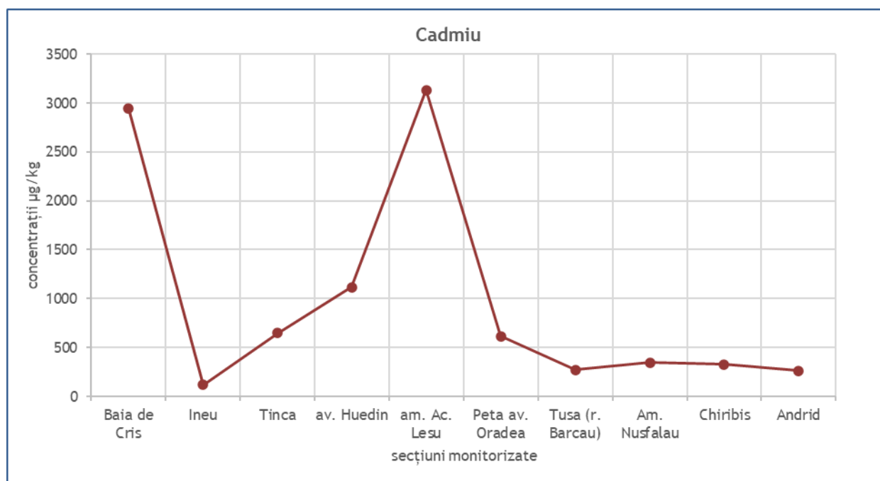
Figura 13 : Variația rezultatelor pentru Cadmiu în secțiunile monitorizate
