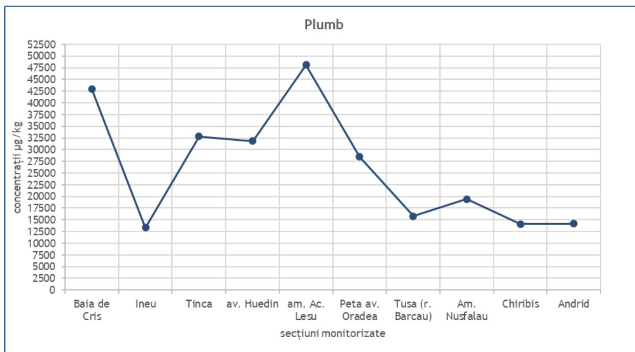
Figura 14 : Variația rezultatelor pentru Plumb în secțiunile monitorizate
