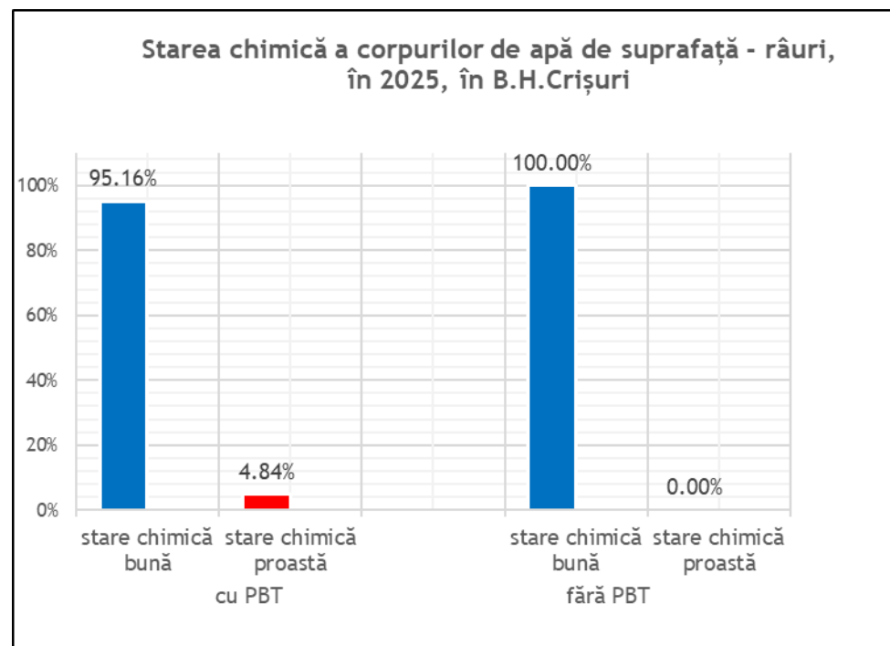
Figura 11 : Starea chimică a corpurilor de apă - râuri în anul 2025
