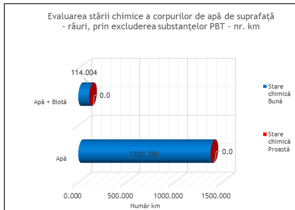
Figura 10 : Evaluarea stării chimice - prin excluderea substanțelor PBT
