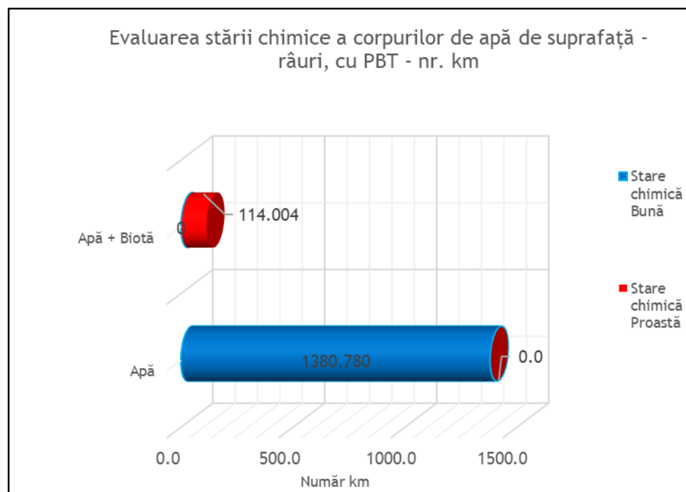
Figura 9 : Evaluarea stării chimice a corpurilor de apă de suprafață - râuri, cu PBT - nr.km
