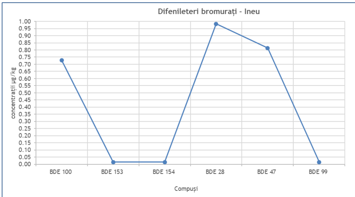
Figura 16 : Variația rezultatelor pentru difenileteri bromurați în secțiunea Ineu
