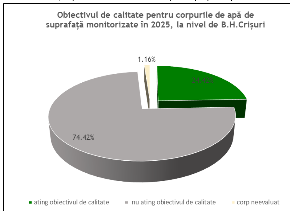
Figura 4 : Situația îndeplinirii obiectivului de calitate pentru corpurile de apă de suprafață - global
